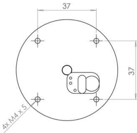
Montagepunkte Leuchtkörper
