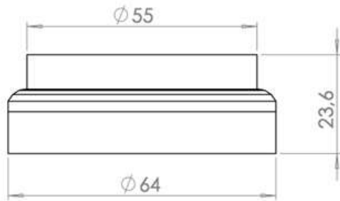
Montagepunkte Leuchtkörper
