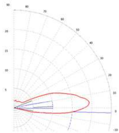
Lichtverteilung
