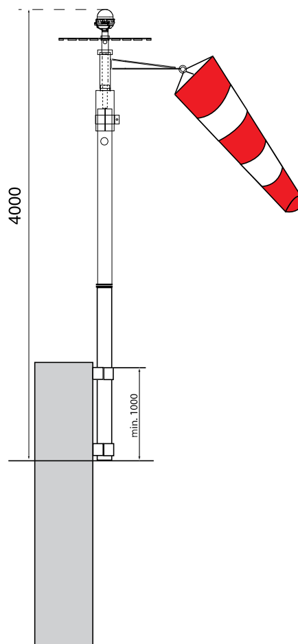
Mât pour montage mural avec éclairage de la manche à vent et feu d'obstacle
